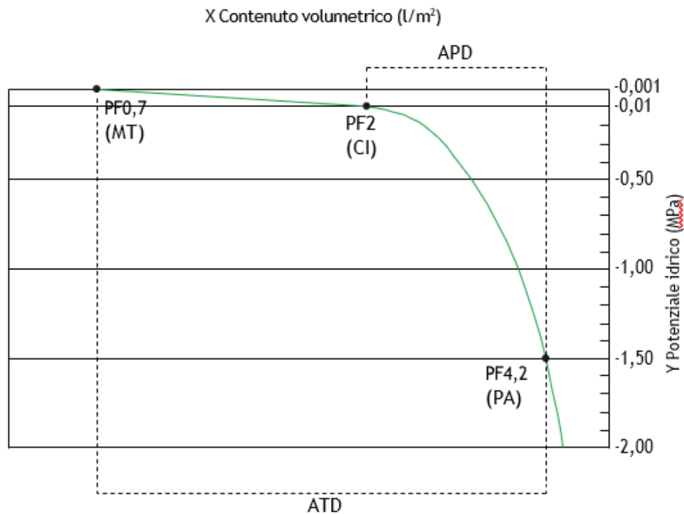
Curva potenziale UNI
